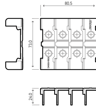
KTB2-10004C
