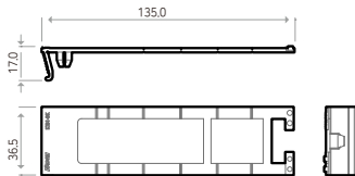
KTB1-BKT
